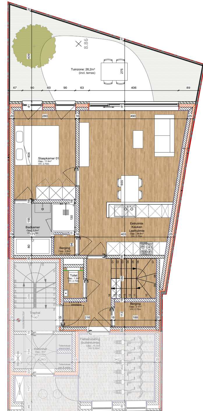
GELIJKVLOERS
